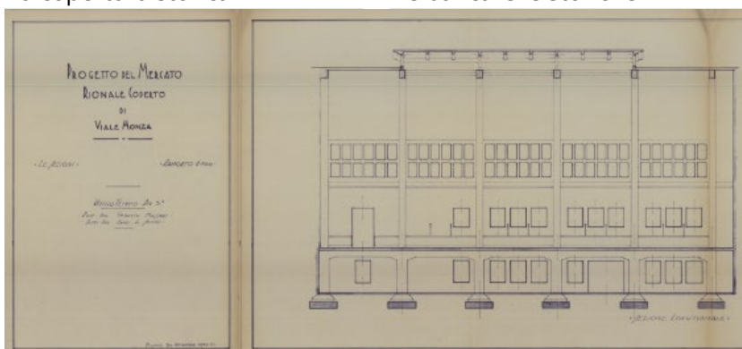
La sezione dell'edificio
